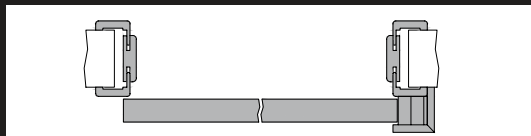
Schiebetür vor der Wand laufend mit Anschlagkasten
