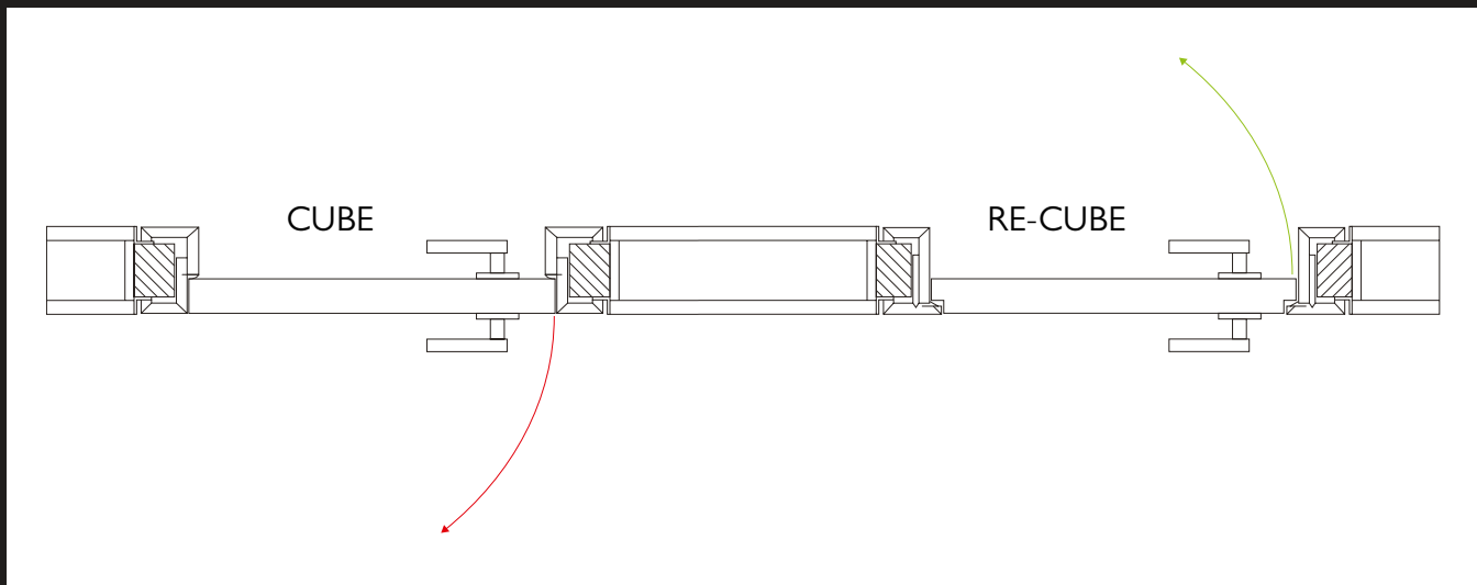
Rot zeigt Standard-CUBE, nach außen zu öffnendes Türblatt. Grün zeigt RE-CUBE, in die Zargen-Leibung zu öffnendes Türblatt.
